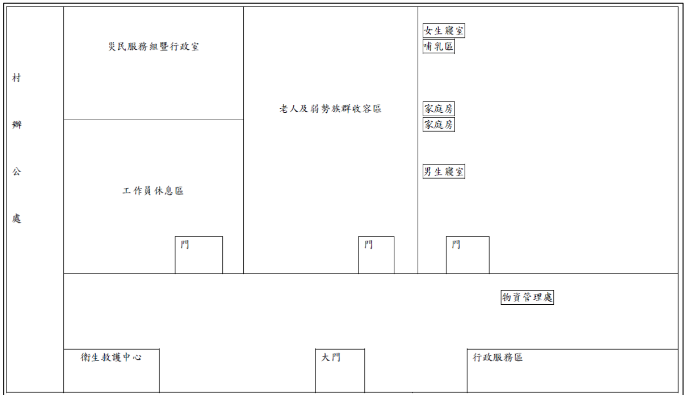
圖 4-2 山中社區活動中心收容空間規劃圖
